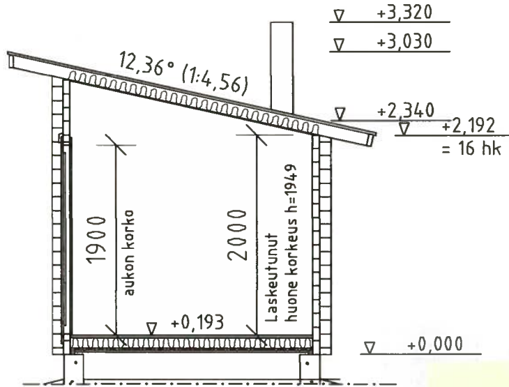
Leikkaus A - A
